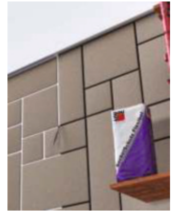
Configurarea îmbinărilor cu lapte de ciment rezistent la apă (ex: protecție flexibilă de brâu Baumit)
